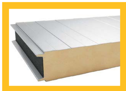
Наполнитель из пенополиуретановой/полиизоциануратной пены (PUR / PIR)
