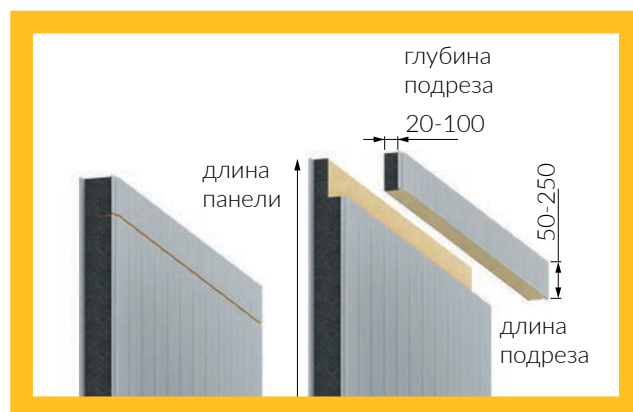
Подрез стеновых панелей.
