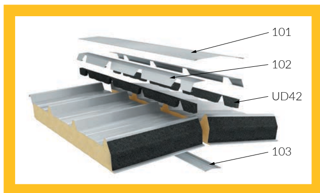
Соединение панелей в конек
